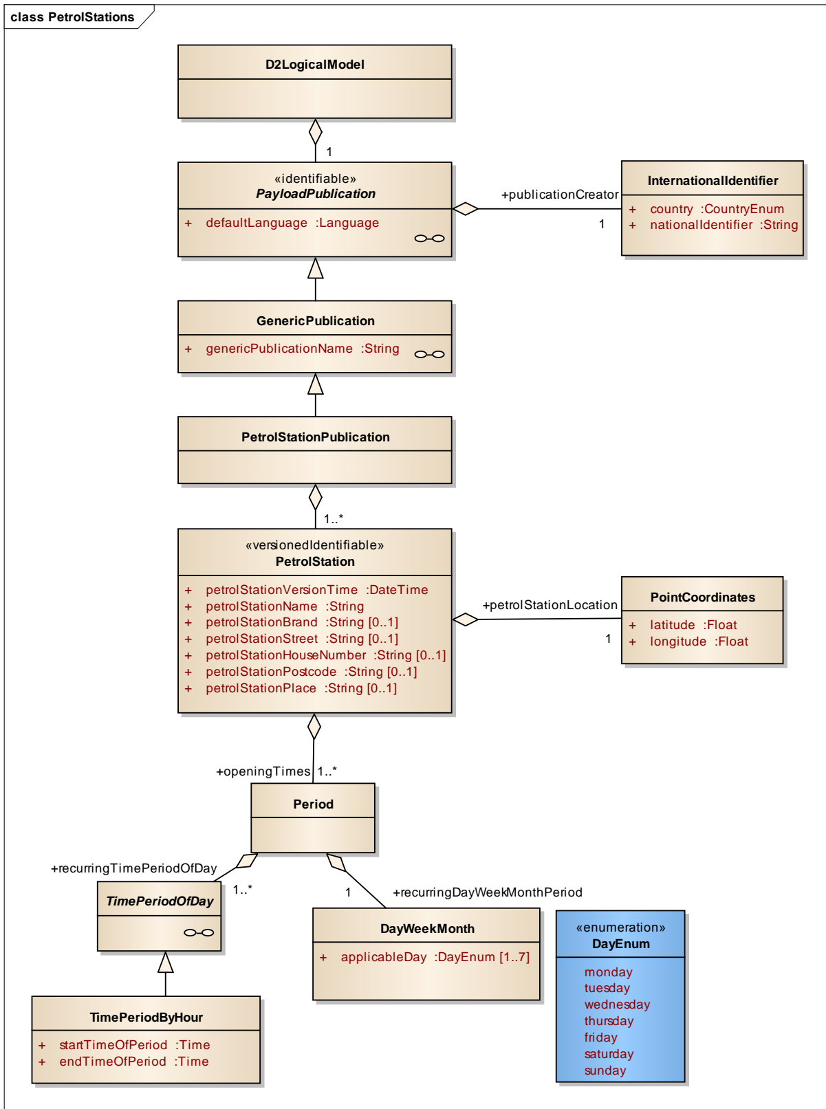
Abbildung 1: Statisches Datenmodell (Grunddaten)
